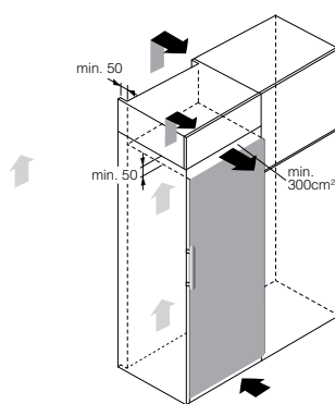
Espace de ventilation
