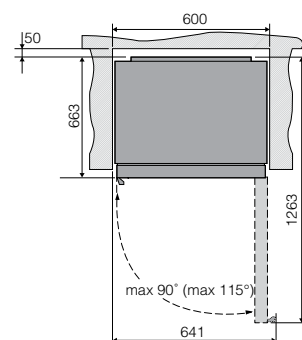
Dimensions encastrement
