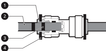
1 Douille de serrage 2 Tuyau 3 Insérer la conduite 4 Clip
